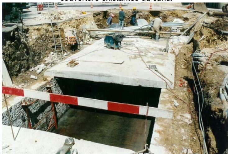
Sciage et enlèvement des dalles de couverture existantes du canal
